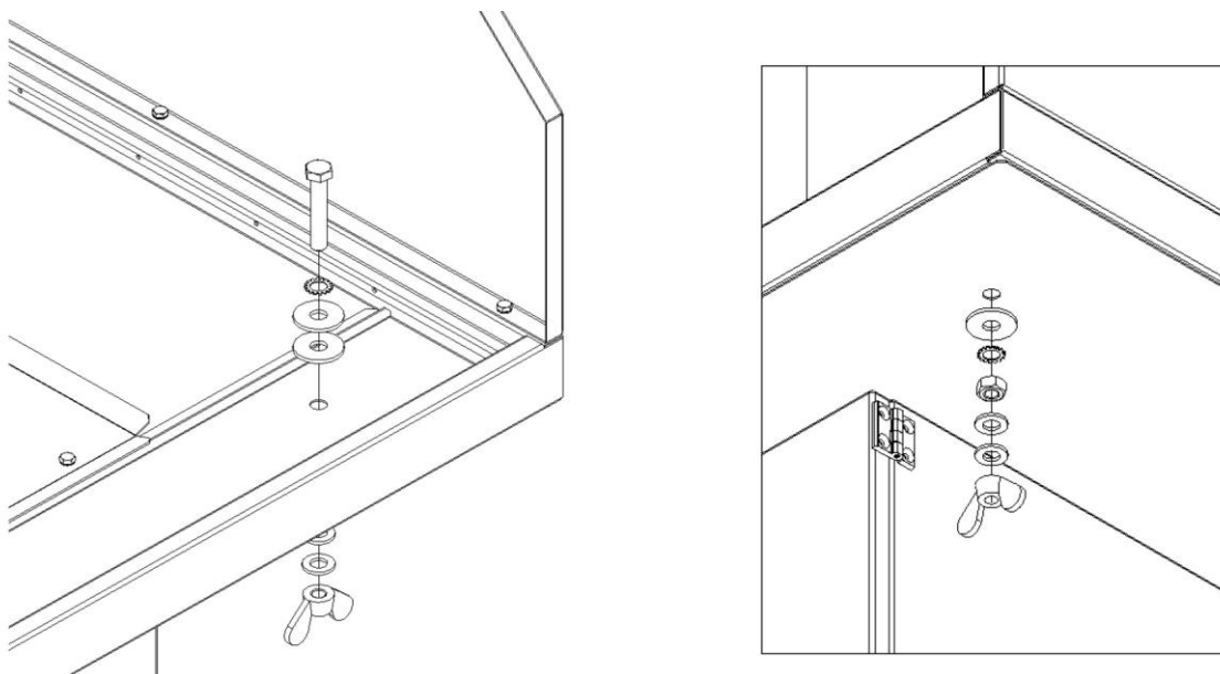
5. ábra: Földelőcsavar felszerelése
