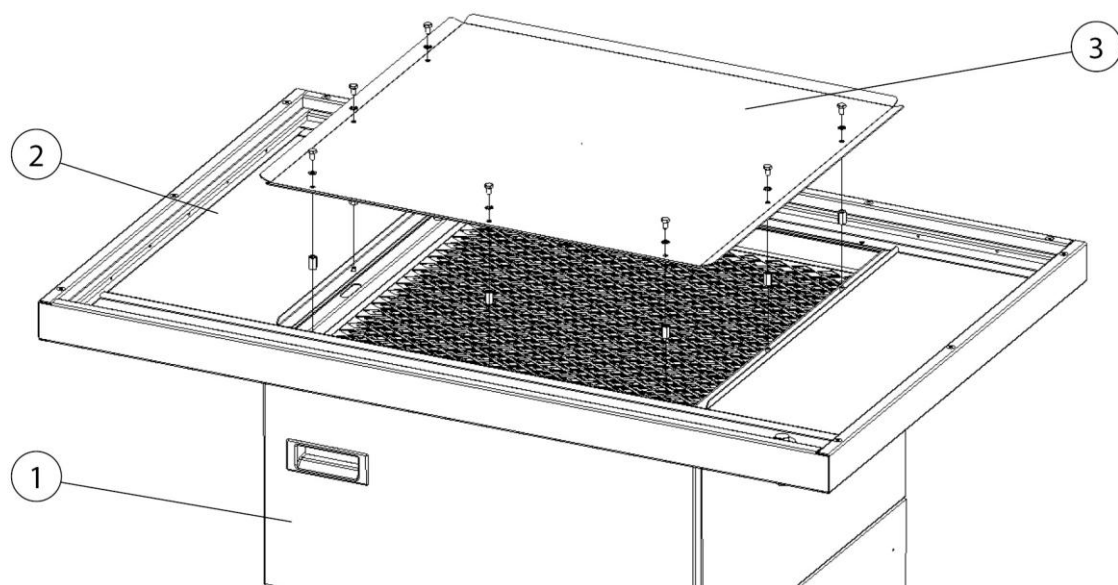
3. ábra: Légtérelő lemez + hegesztési asztal felszerelése
