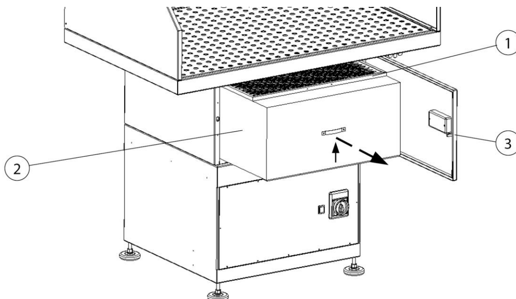
10. ábra: Szűrőcsere - Előszűrő + Főszűrő
