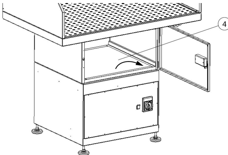
11. ábra: Szűrőcsere - Aktivszén-szűrő (opcionális)
