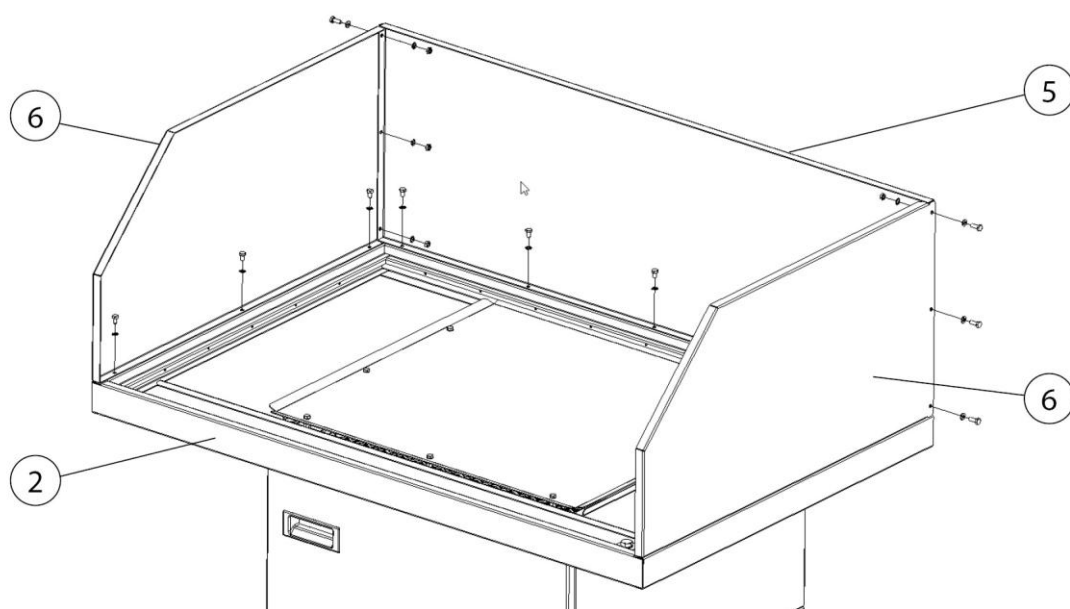
4. ábra: Oldalfalak + hátfal felszerelése
